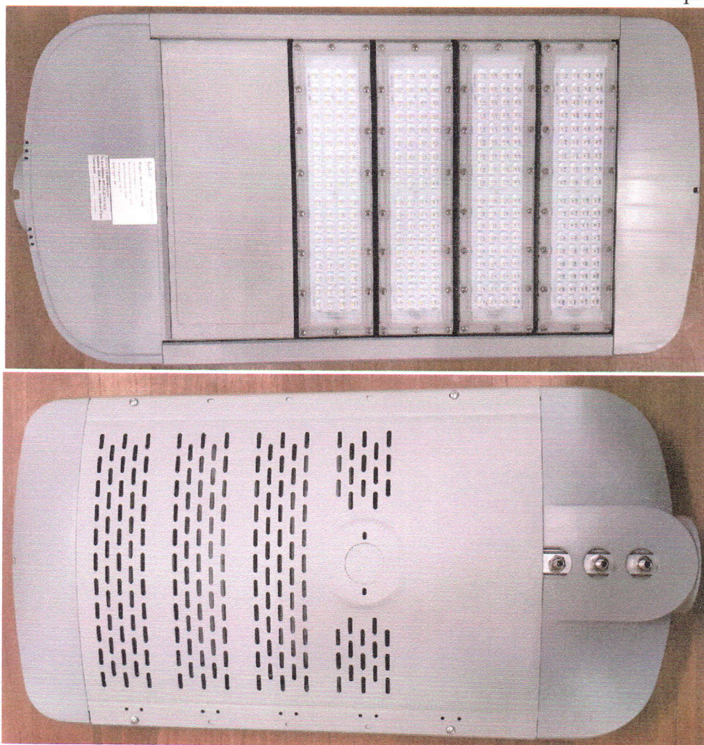
Рисунок 3 – Фотографии образца светильник светодиодный PCcooler BP-001-0018 (120Вт)
