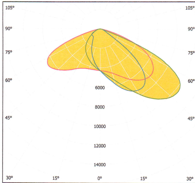
Рисунок 1 – КСС образца светильник светодиодный РС cooler ВР-001-0018 (120Вт) в поперечной (С0-С180) (красная кривая), продольной (С90-С270) (синяя кривая) плоскостях и плоскости максимальной силы света (С30-С210) (зеленая кривая)
